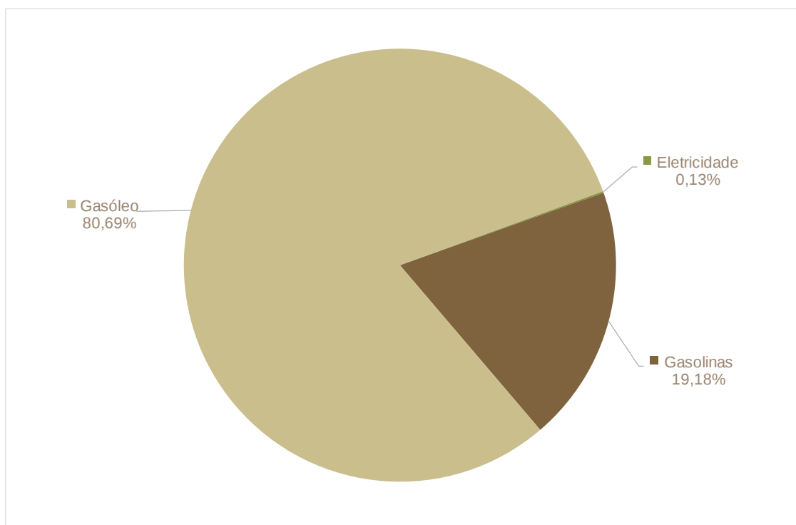
Figura 48: Emissões de CO 2 no setor dos transportes no Município de Castelo de Vide por vetor energético [%]
