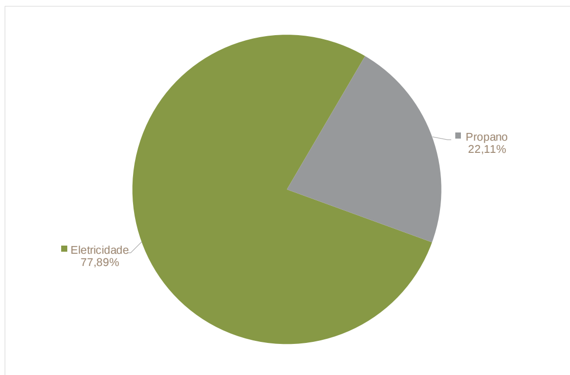
Figura 44: Emissões de CO 2 no setor de serviços no Município de Castelo de Vide por vetor energético [%]
