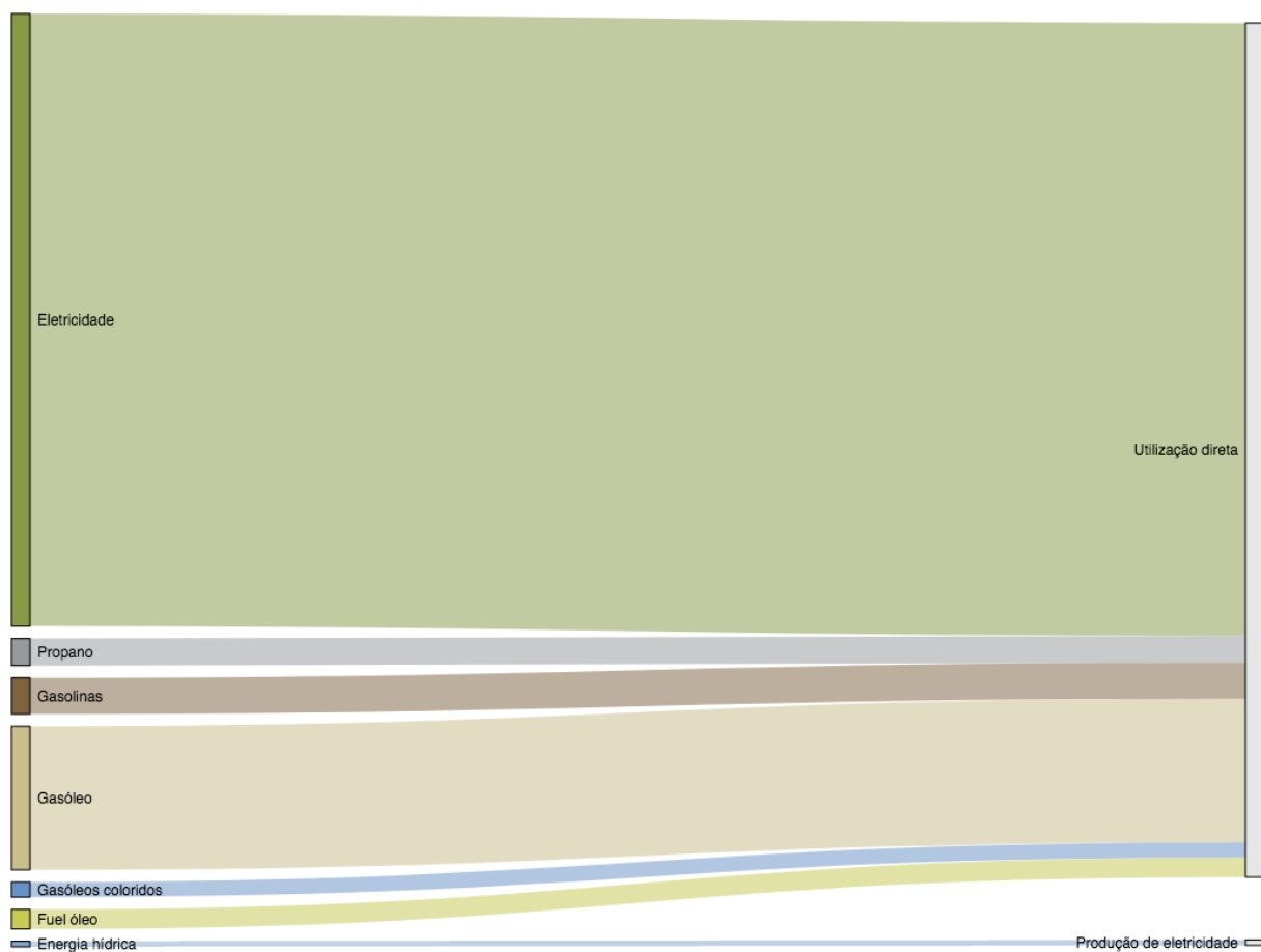
Figura 36: Diagrama de Sankey da utilização de fontes de energia primária no Município de Castelo de Vide
