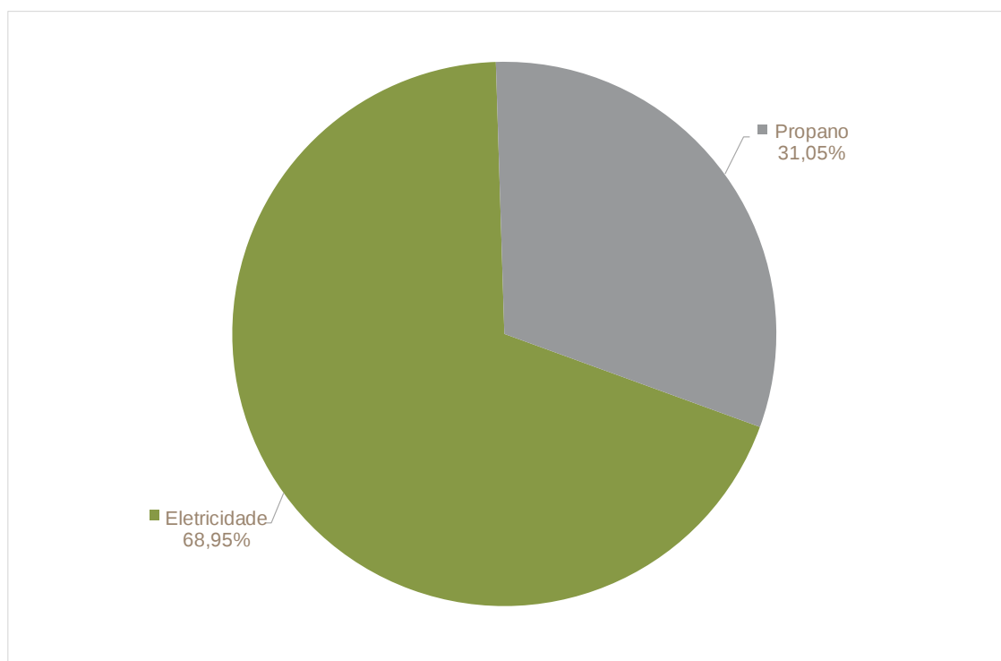
Figura 43: Utilização de energia final no setor de serviços no Município de Castelo de Vide por vetor energético [%]
