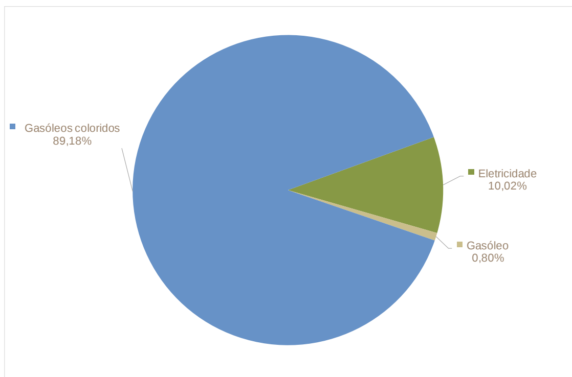
Figura 65: Utilização de energia final no setor da agricultura e pescas no Município de Castelo de Vide por vetor energético [%]
