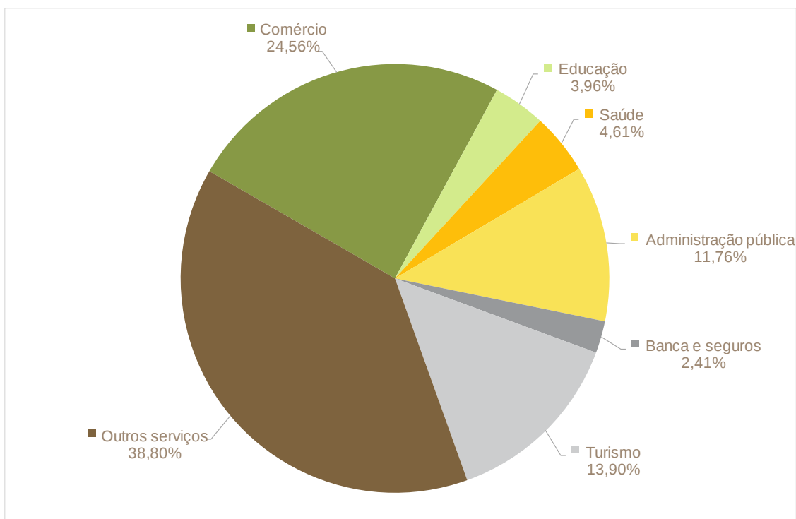
Figura 13: Emissões de CO 2 em serviços em Portugal por agrupamento de atividade económica [%]
