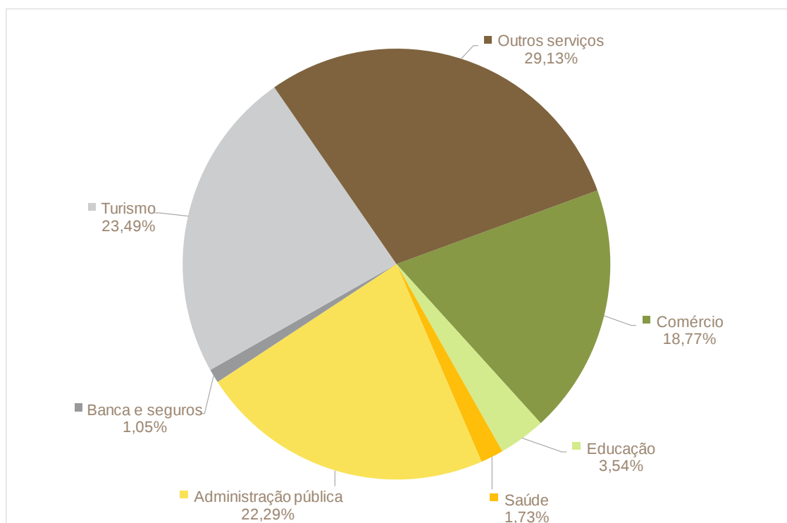
Figura 46: Emissões de CO 2 em serviços no Município de Castelo de Vide por agrupamento de atividade económica [%]
