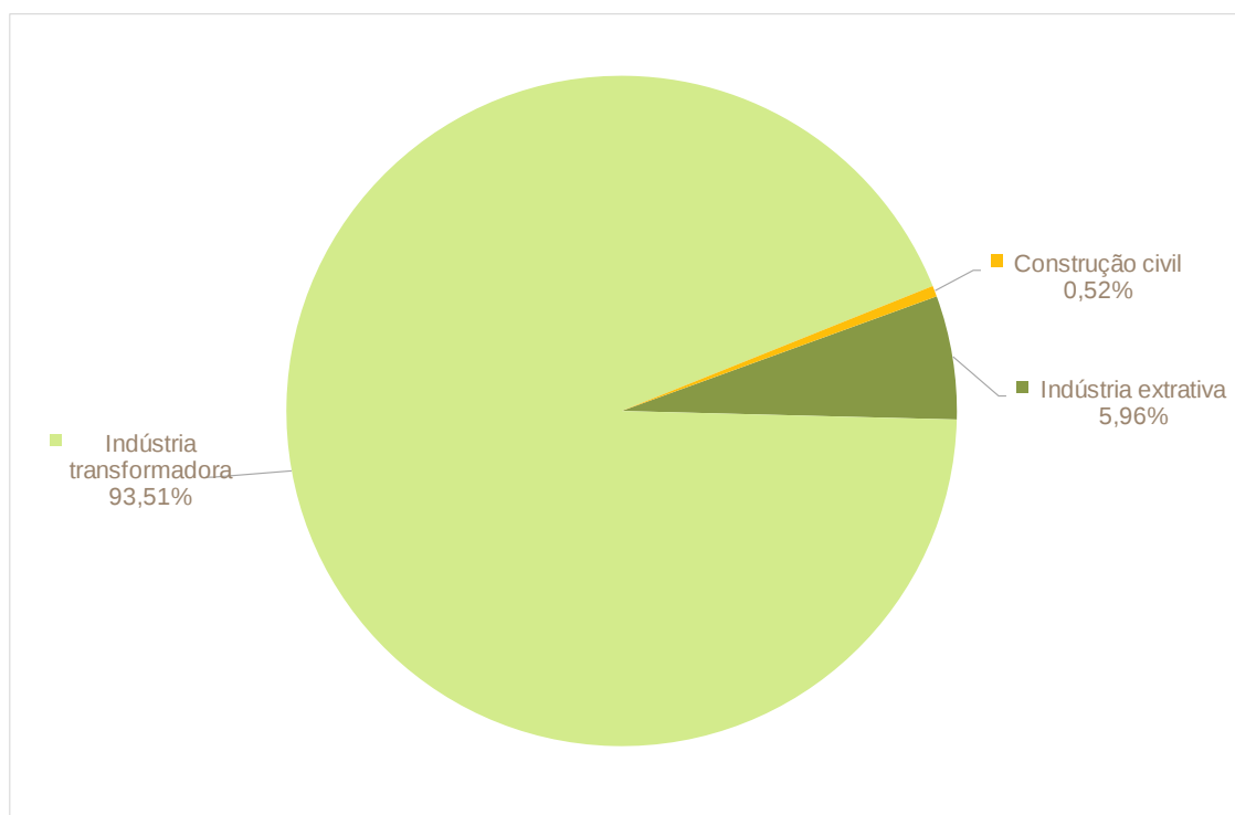
Figura 56: Emissões de CO 2 na indústria no Município de Castelo de Vide por subsetor de atividade [%]
