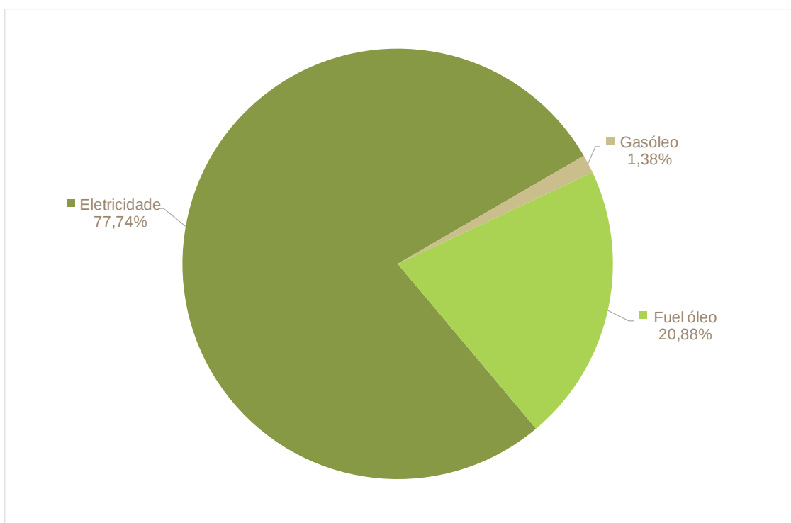
Figura 59: Utilização de energia final na indústria transformadora no Município de Castelo de Vide por vetor energético [%]
