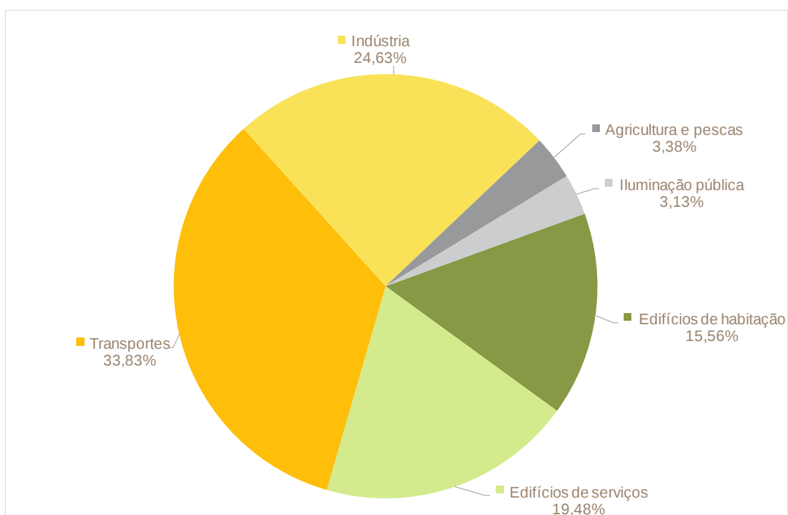
Figura 40: Emissões de CO 2 no Município de Castelo de Vide por setor consumidor de energia [%]
