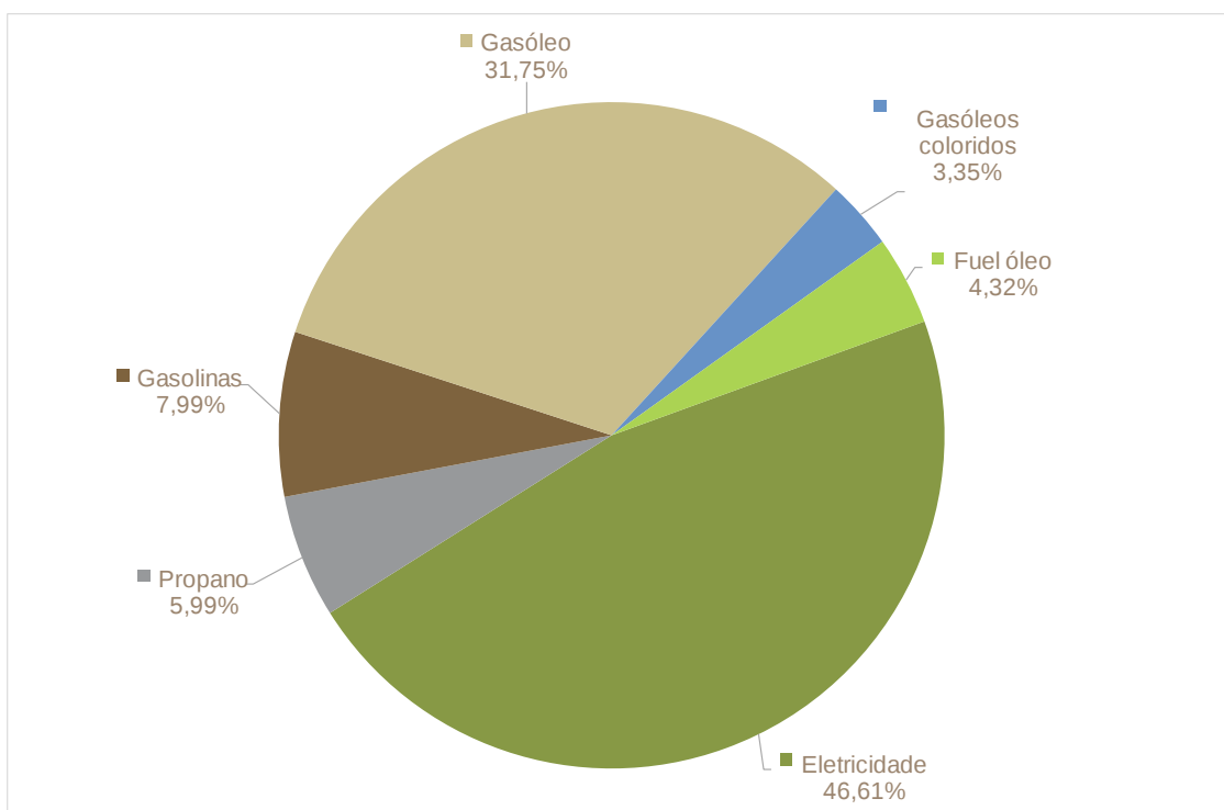
Figura 37: Utilização de energia final no Município de Castelo de Vide por vetor energético [%]
