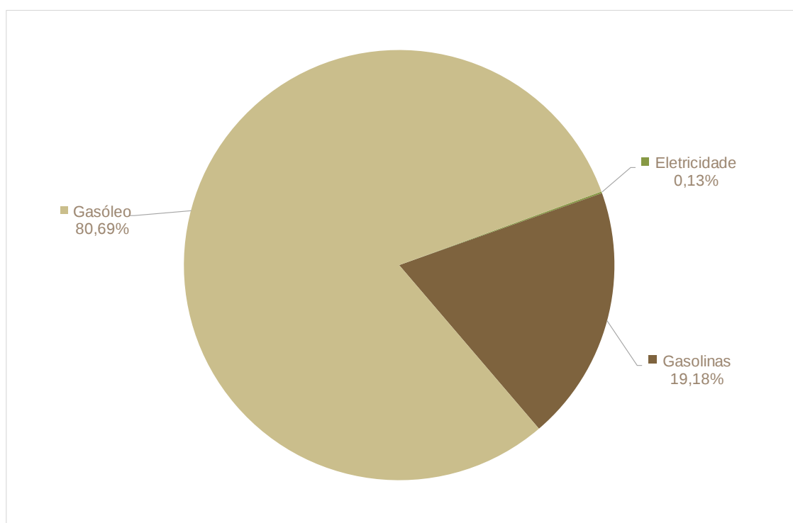
Figura 50: Emissões de CO 2 no subsetor transportes privados no Município de Castelo de Vide por vetor energético [%]
