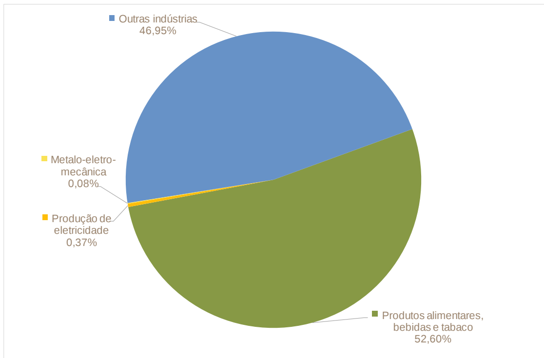
Figura 61: Utilização de energia final na indústria transformadora no Município de Castelo de Vide por agrupamento de atividade económica [%]
