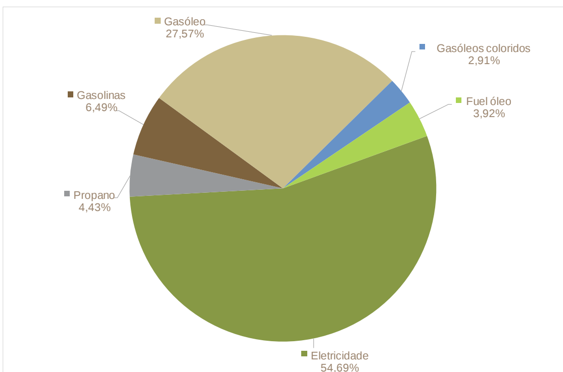
Figura 38: Emissões de CO 2 no Município de Castelo de Vide por vetor energético [%]
