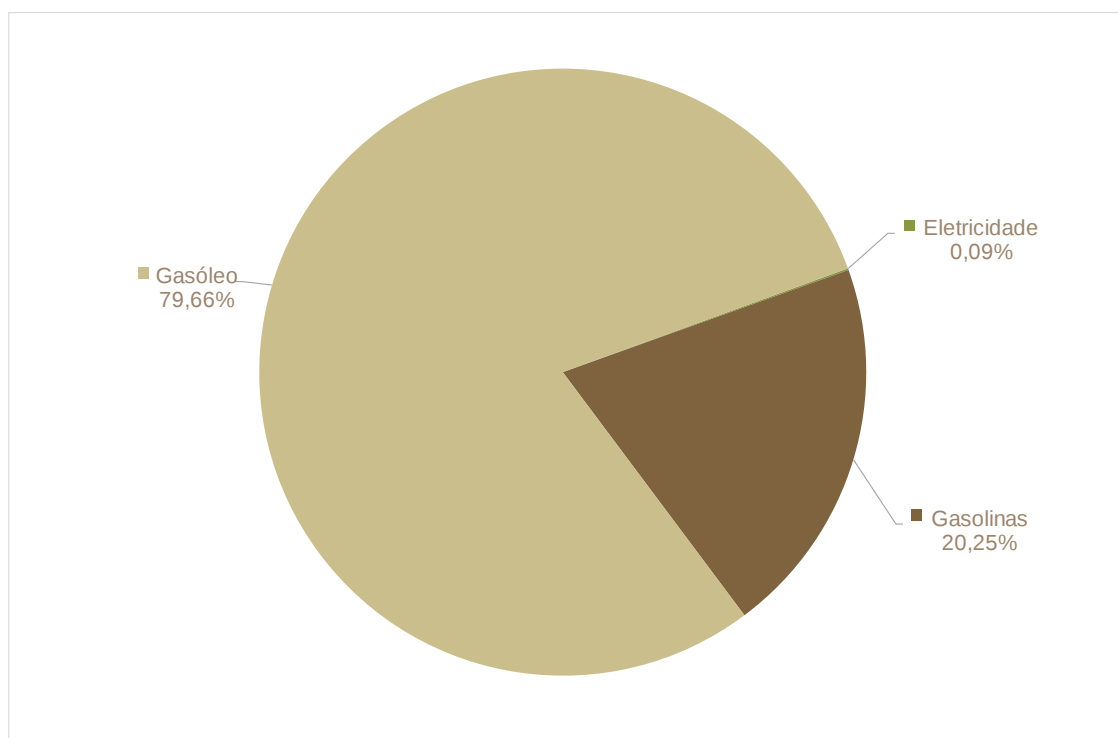
Figura 49: Utilização de energia final no subsetor transportes privados no Município de Castelo de Vide por vetor energético [%]
