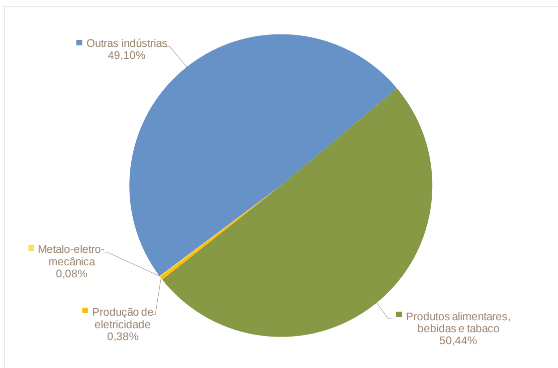
Figura 62: Emissões de CO 2 na indústria transformadora no Município de Castelo de Vide por agrupamento de atividade económica [%]
