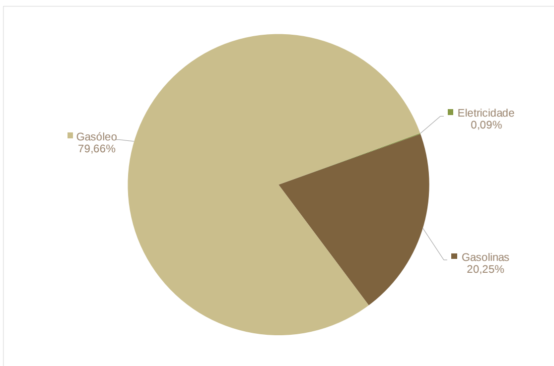
Figura 47: Utilização de energia final no setor dos transportes no Município de Castelo de Vide por vetor energético [%]
