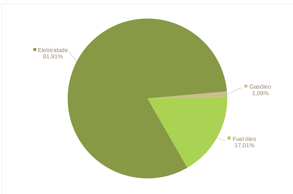
Figura 60: Emissões de CO 2 na indústria transformadora no Município de Castelo de Vide por vetor energético [%]
