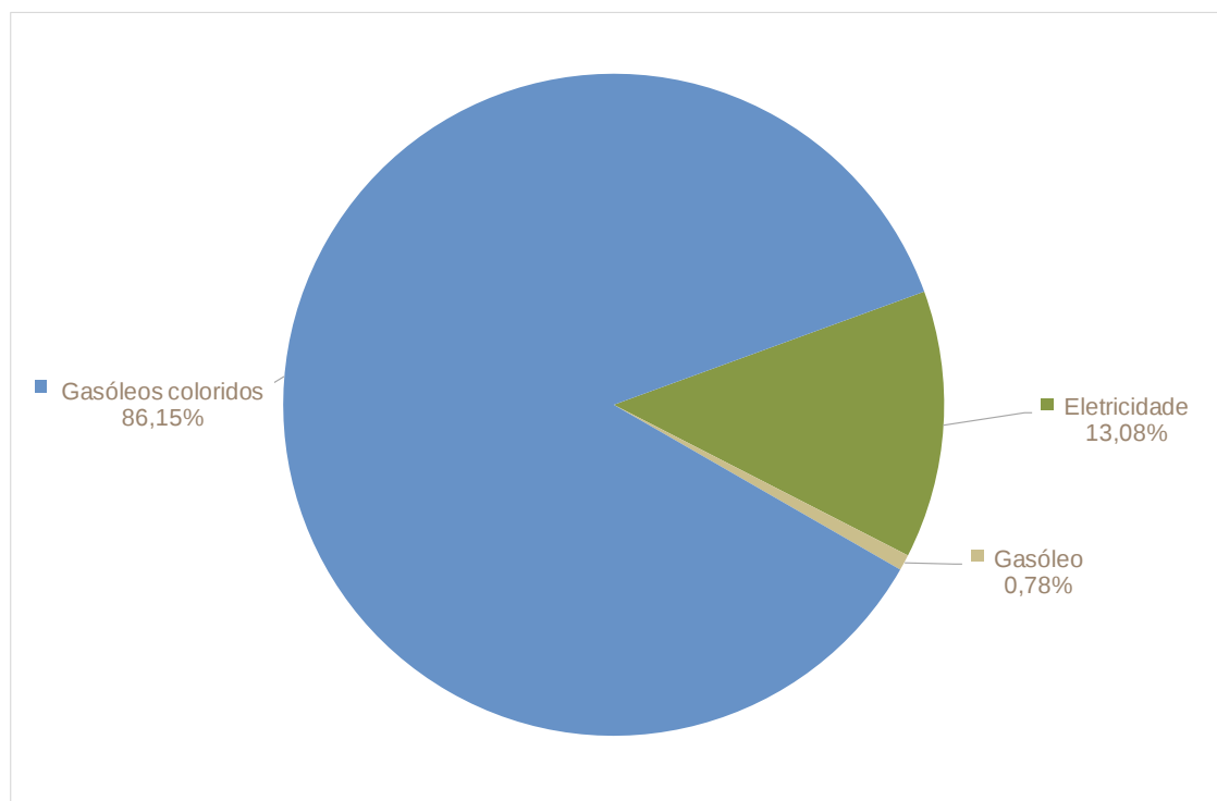
Figura 66: Emissões de CO 2 no setor da agricultura e pescas no Município de Castelo de Vide por vetor energético [%]
