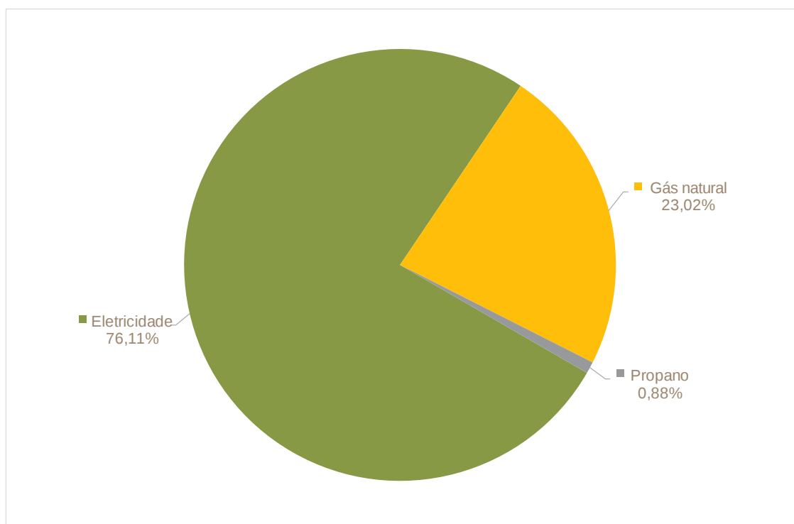
Figura 43: Utilização de energia final no setor de serviços no Município de Campo Maior por vetor energético [%]
