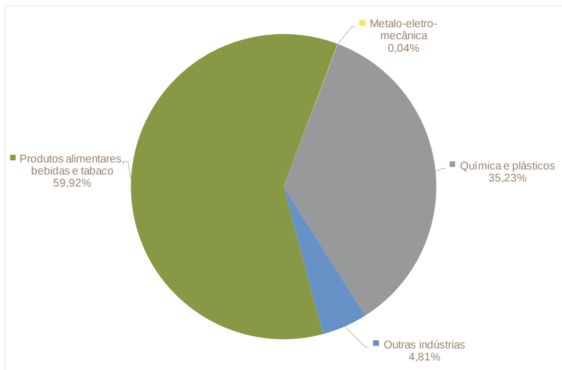
Figura 63: Utilização de energia final na indústria transformadora no Município de Campo Maior por agrupamento de atividade económica [%]
