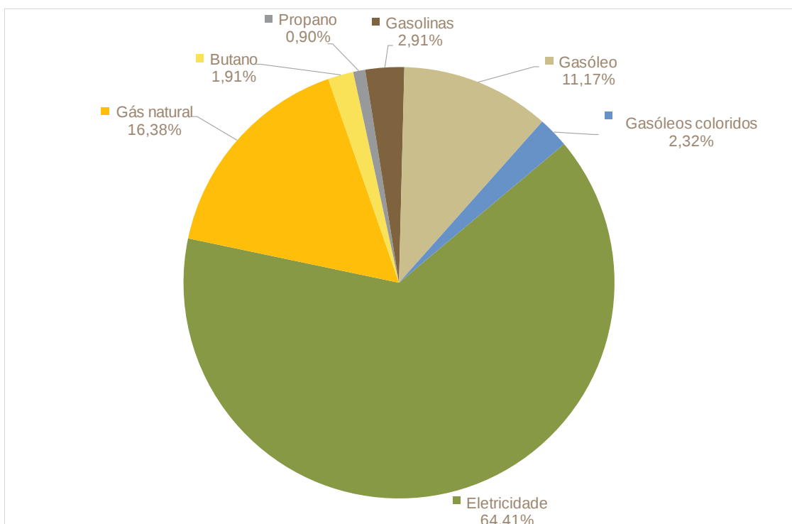
Figura 35: Emissões de CO 2 no Município de Campo Maior por vetor energético primário [%]
