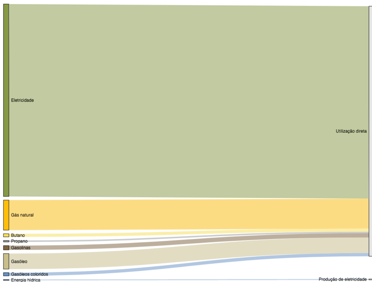
Figura 36: Diagrama de Sankey da utilização de fontes de energia primária no Município de Campo Maior
