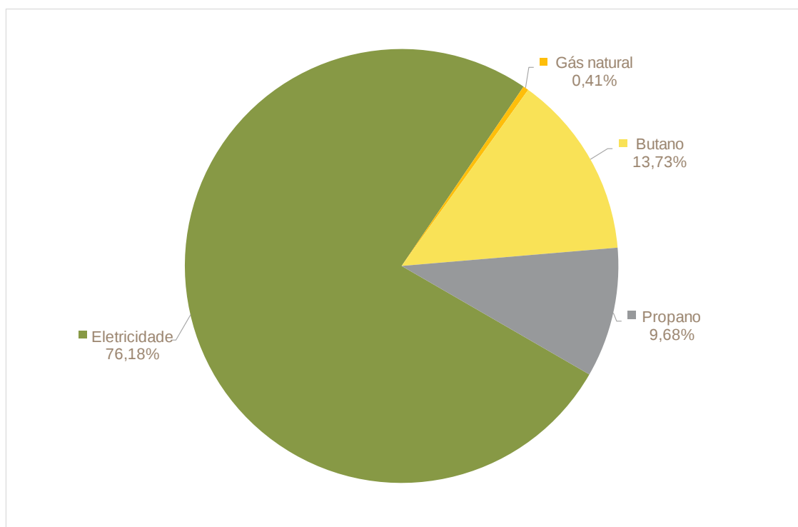
Figura 41: Utilização de energia final no setor residencial no Município de Avis por vetor energético [%]
