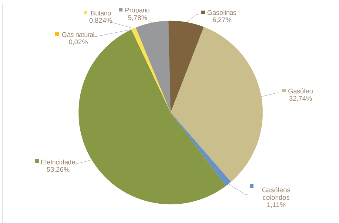
Figura 35: Emissões de CO 2 no Município de Avis por vetor energético primário [%]
