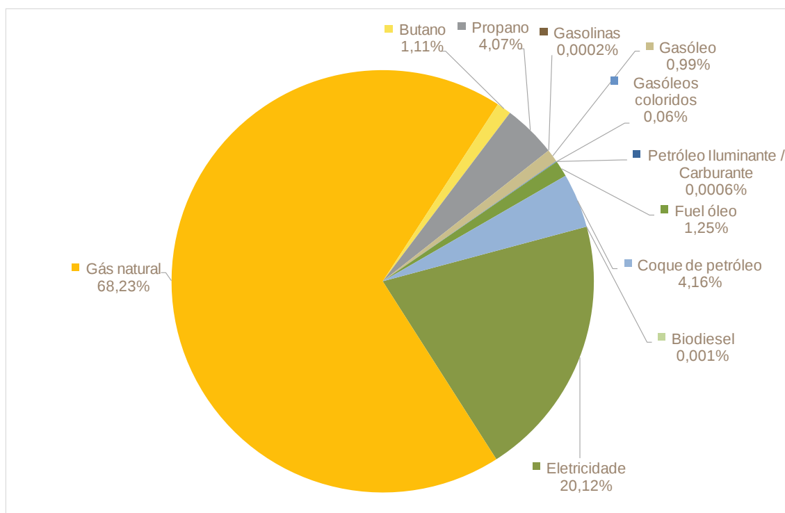
Figura 22: Utilização de energia final na indústria transformadora em Portugal por vetor energético [%]
