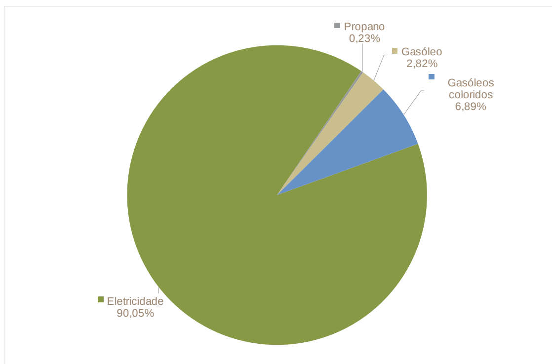
Figura 67: Utilização de energia final no setor da agricultura e pescas no Município de Avis por vetor energético [%]
