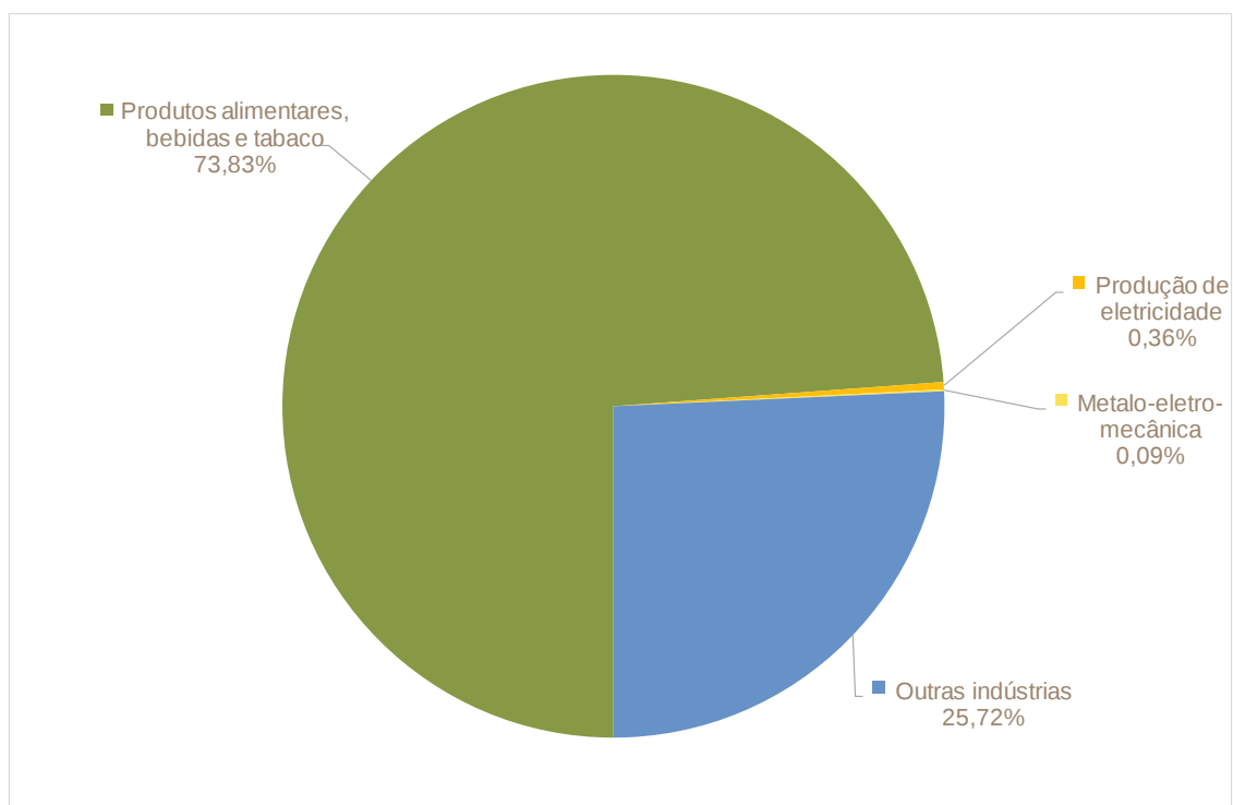
Figura 64: Emissões de CO 2 na indústria transformadora no Município de Avis por agrupamento de atividade económica [%]
